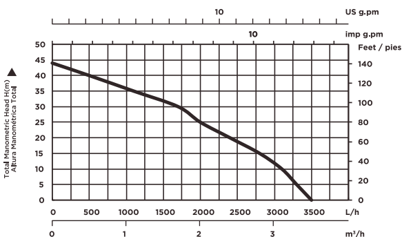
PERFORMANCE CURVE - CURVA DE EFICIENCIA
