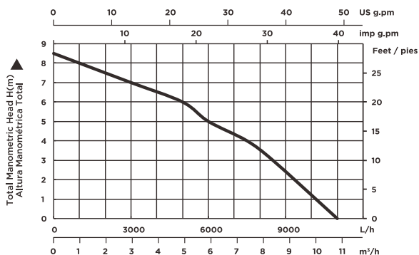
PERFORMANCE CURVE - CURVA DE EFICIENCIA
